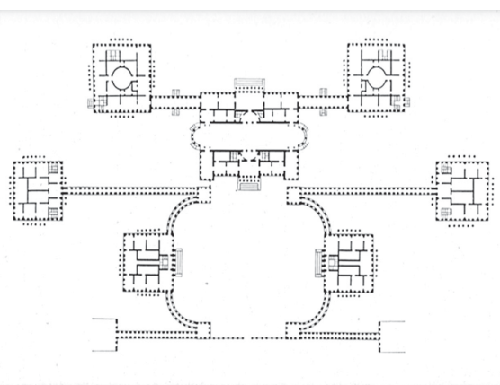
План дворцового ансамбля в Пелле. Из собрания чертежей Кваренги в Академии Каррара в Бергамо (Италия)
